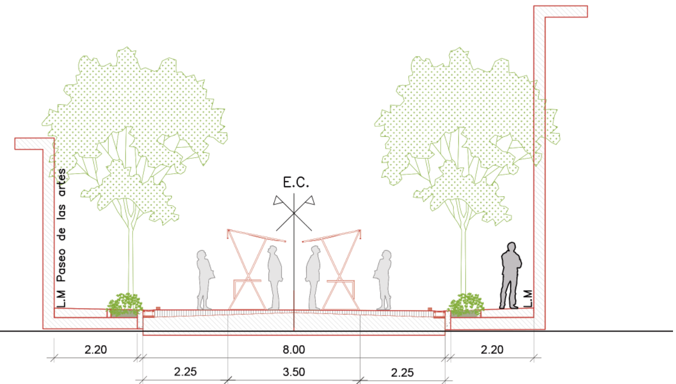
PERFIL CALLE LAPRIDA PROPUESTA
