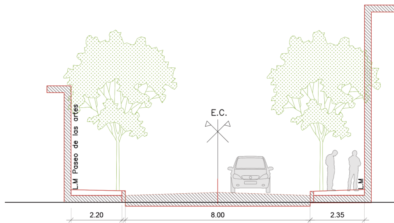
PERFIL CALLE LAPRIDA EXISTENTE
